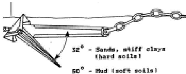
STATO Anchor
