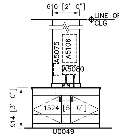
① U0049 ELEVATION
