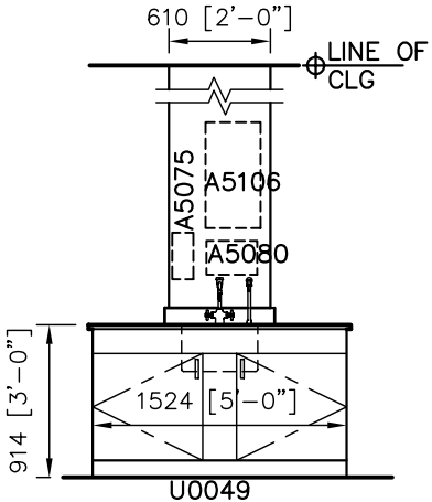
① U0049 ELEVATION
