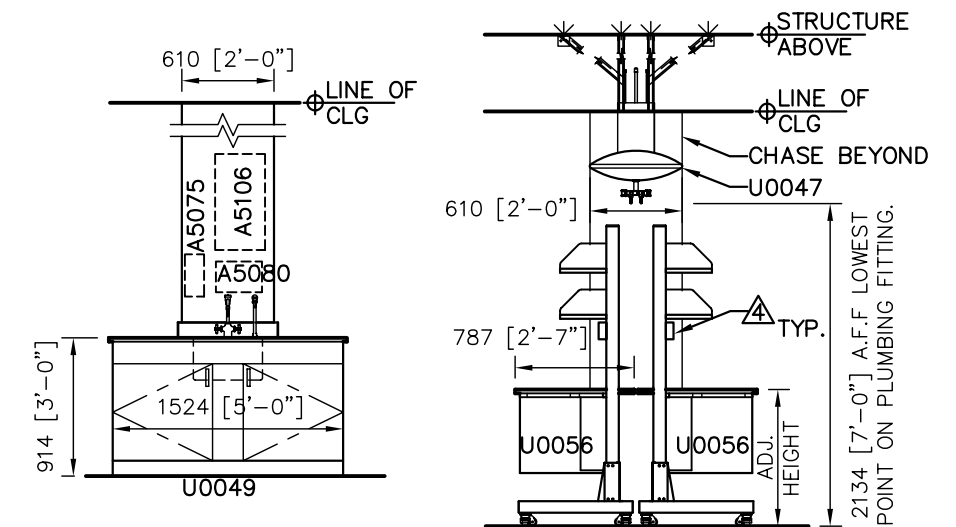
① U0049 ELEVATION
