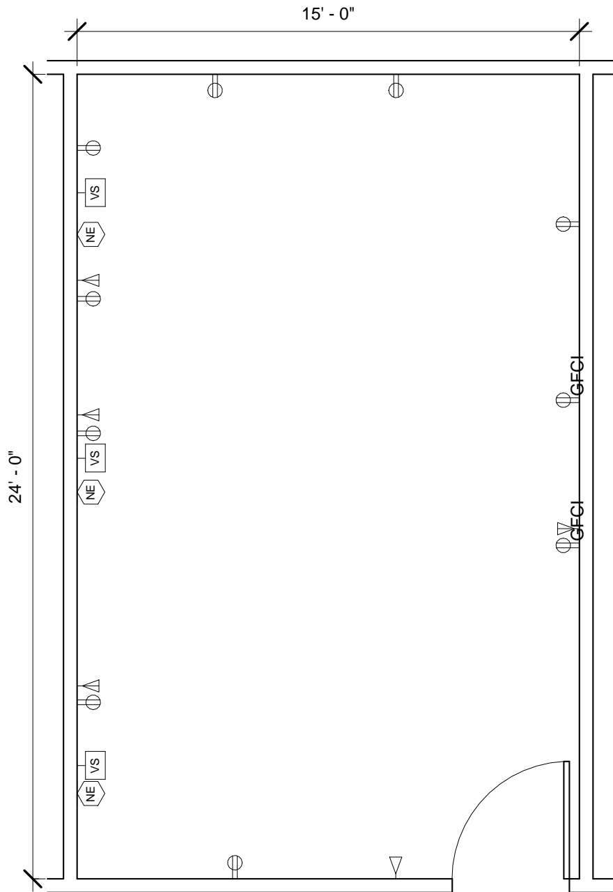
OPRT1 - FLOOR PLAN
